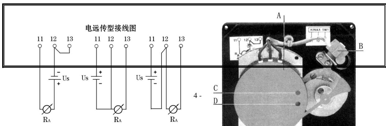
转角变送器接线图
